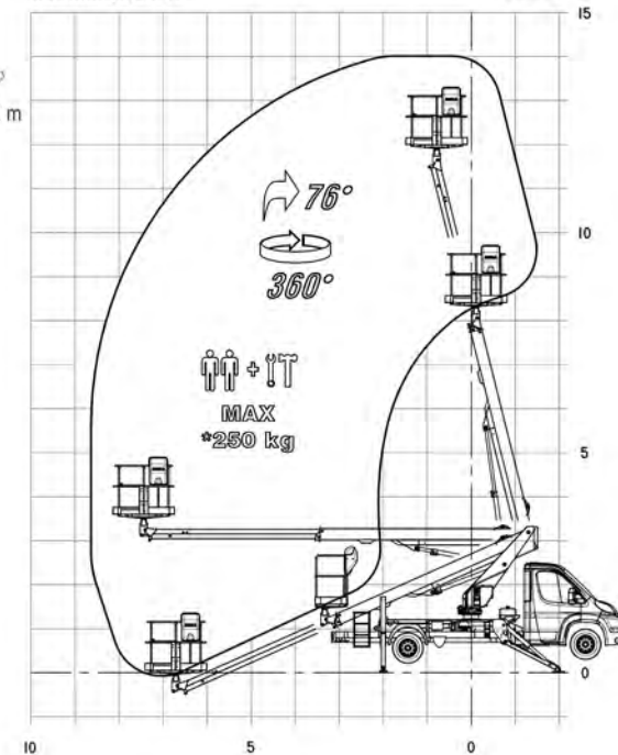
DIAGRAMMA DI LAVORO WORKING DIAGRAM
